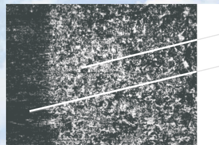
Структура листового титанового сплава ОТ4-1 толщиной 2 мм после лазерного отжига: 1 – зона отжига; 2 – исходная структура
