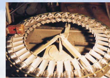
Нанесение турбинных лопаток в колесе на специальном оборудовании
