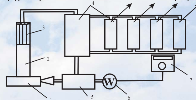
1 - система закрутки потока; 2 - кавитационная труба; 3 - развихритель; 4 - теплопередающие устройства (теплообменник, батареи, calorifiers); 5 - гидронасос; 6 - электродвигатель; 7 - пульт управления работой теплогенератора
