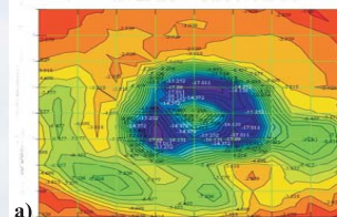
Поле осевой скорости W_x капель в топливно-воздушном факеле пневмомеханической форсунки ГТД: а – изображение в 2D; б – изображение в 3D
