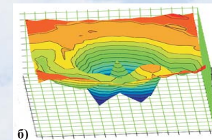
Поле осевой скорости W_x капель в топливно-воздушном факеле пневмомеханической форсунки ГТД: а – изображение в 2D; б – изображение в 3D
