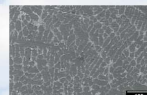
С магнитно-импульсной обработкой (W=0,56 кДж, n=3 имп.)
