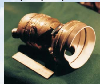
Труба жаровая двигателя НК-36СТ с теплозащитным металлокерамическим покрытием
