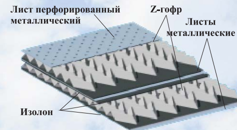
Акустическая панель с заполнителем в виде Z-гофра
