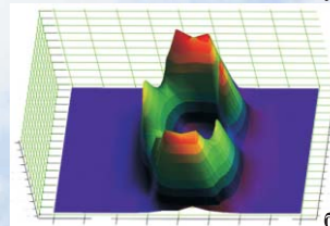
Поле распределения массы жидкого топлива в топливно-воздушном факеле форсунки ГТД: а – изображение в 2D; б – изображение в 3D
