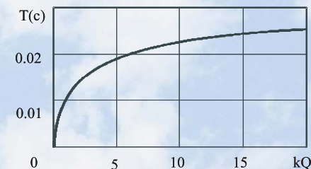
Зависимость времени растекания жидкости от степени чистоты и шероховатости поверхности
