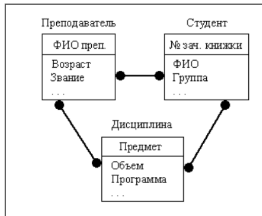
Рис. 1. Фрагмент IDEF1X-модели
