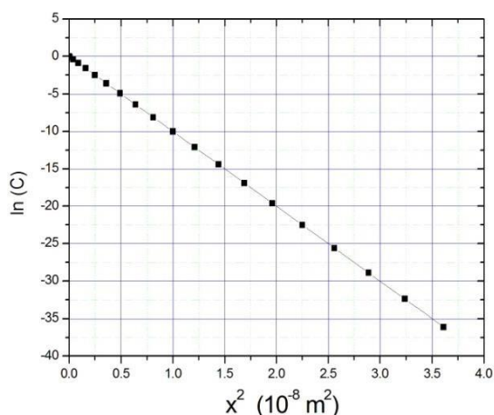
Рис.2: Диффузионный профиль для элемента А в В перестроенный в координатах \ln C vs. x^2 .
