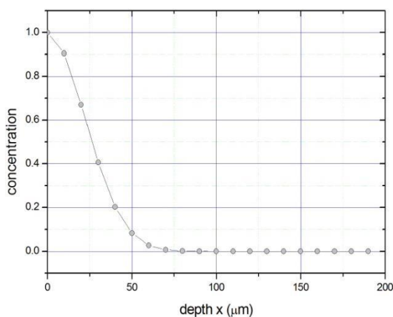
Рис.1: Измеренный профиль концентрации, C (в произвольных единицах) для диффузии элемента А в В. x - глубина в микрометрах
