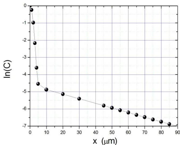
Рис. 3: Концентрационный профиль померянный во втором эксперименте для диффузии элемента А в материале В, построенный в координатах логарифм концентрации - глубина.
