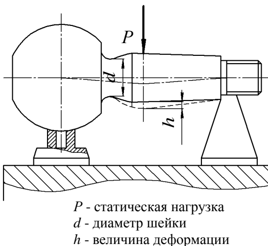
Рисунок 1 – Проверка прочности шарового пальца
